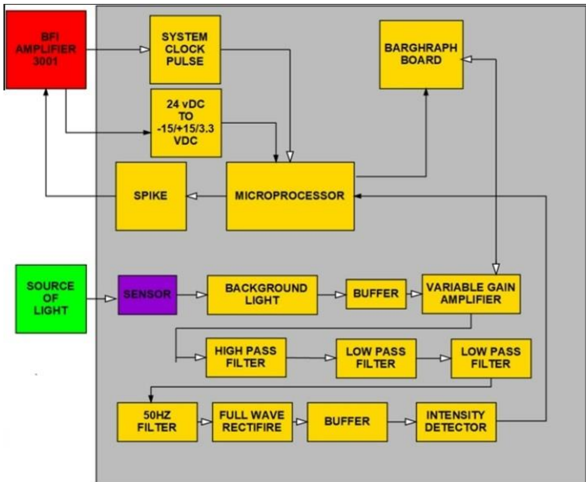
بلوک دیاگرام فلیم اسکنر (Flame Scanner)
